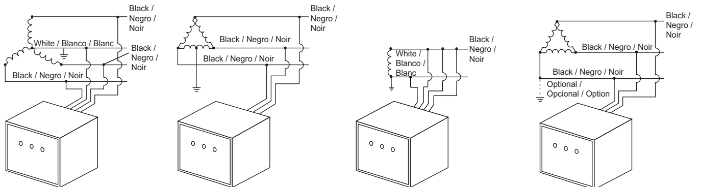
3-Phase, 4-Wire WYE 3 fases, 4 hilos en estrella trifasée, 4 fils en étoile
